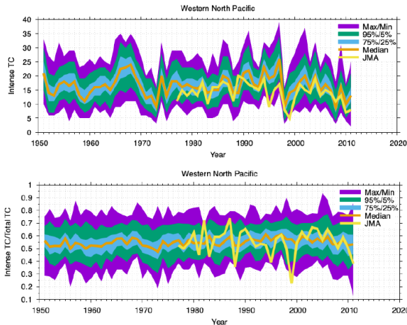
上：発生数、下：強い台風の割合。黄色が観測値（気象庁ベストトラック）
