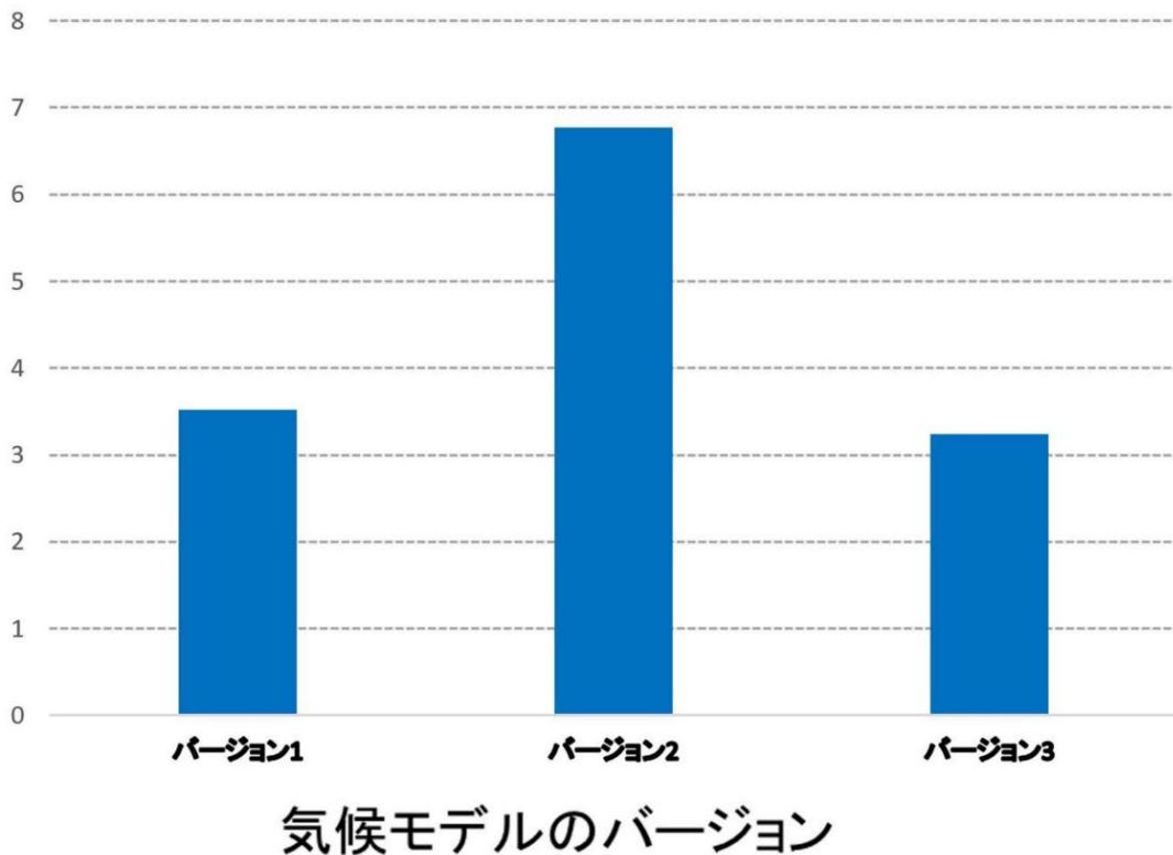
図 48ドイツの研究グループのモデル。バージョン1は2013年のIPCC予測に使われたモデルだった。だがそのバグを取ったらバージョン2のように気温上昇が倍になってしまった。その後気温上昇が3°Cになる様に雲のパラメーターを調整して、今はバージョン3のモデルを予測に使用している。(Mauritsen & Roeckner, 2020)のFigure 2を元に筆者作成。
