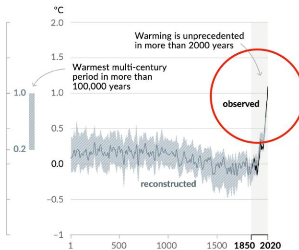
図 7 IPCC AR6 WG1 Figure SPM.1 Presentation の抜粋(スライド 4。出典:IPCC [6])
