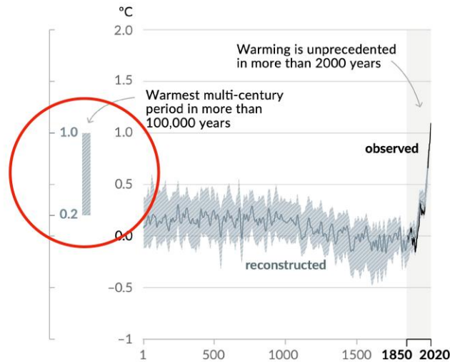
図8 IPCC AR6 WG1 Figure SPM.1 Presentation の抜粋(スライド5。出典:IPCC [6])
